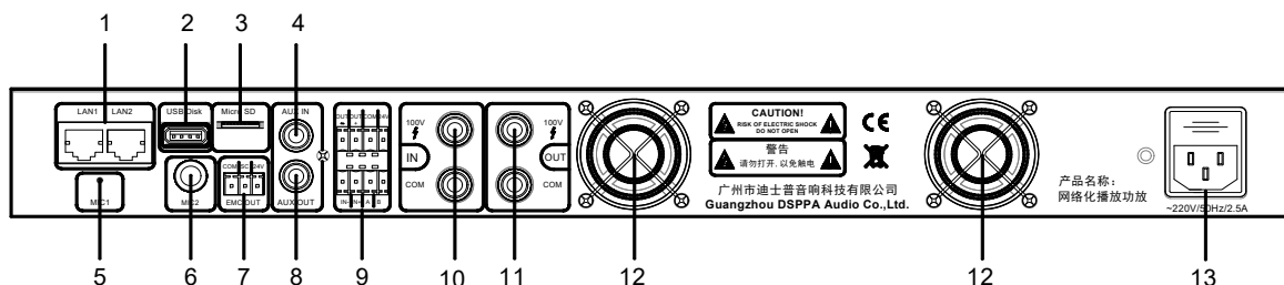
MAG6825/MAG6835/MAG6850/MAG6865 Rear Panel
